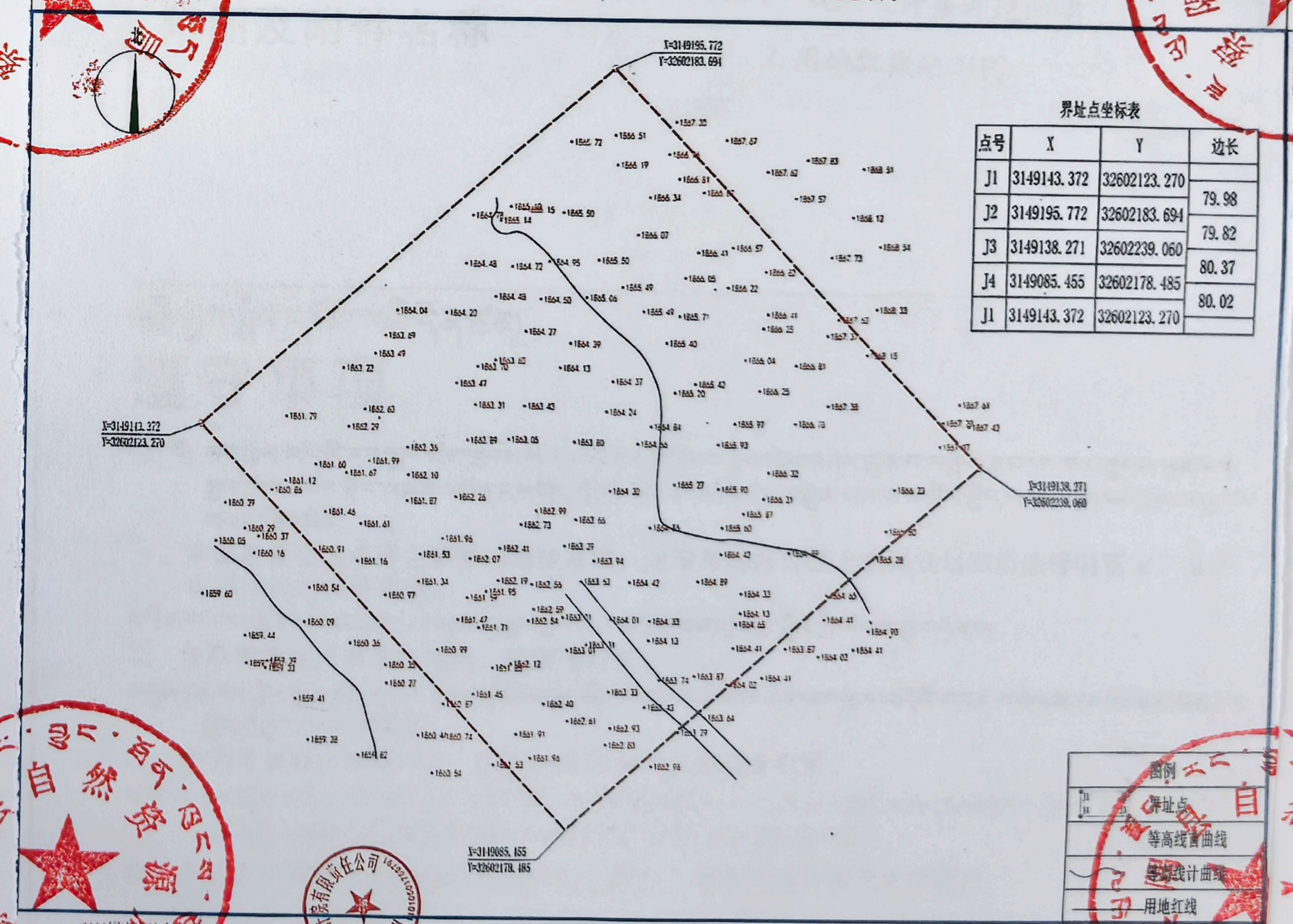
林芝市察隅县喀仁混凝土有限公司商混站建设项目一用地地形图
