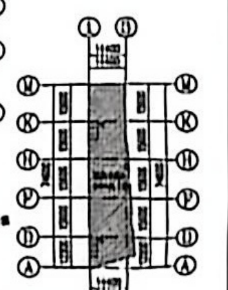
三层平面防火分区示意图 1:1000 比例尺: 1:1000
