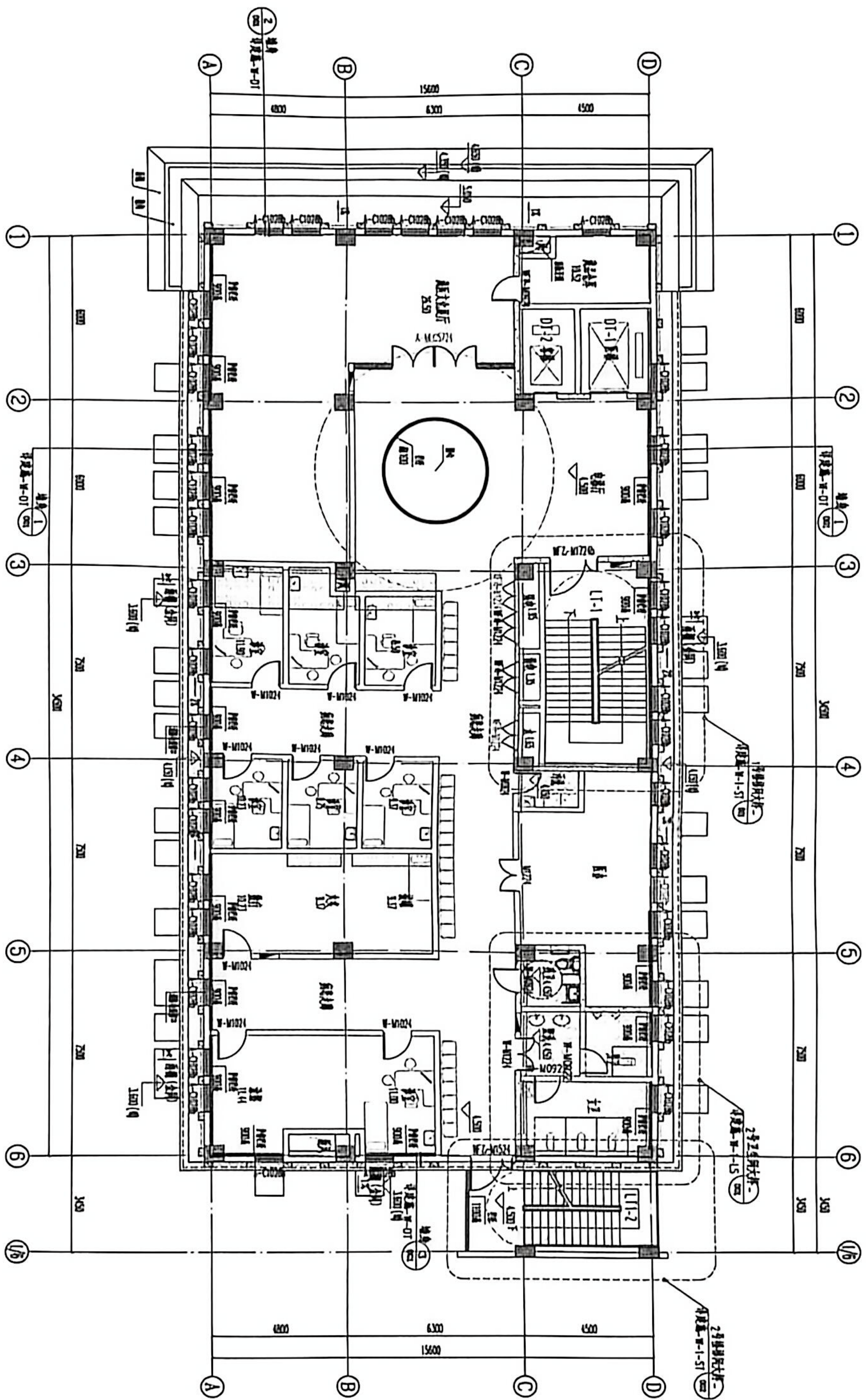
建筑二层平面图 比例尺 1:100 本图依据GB50485-2019标准
